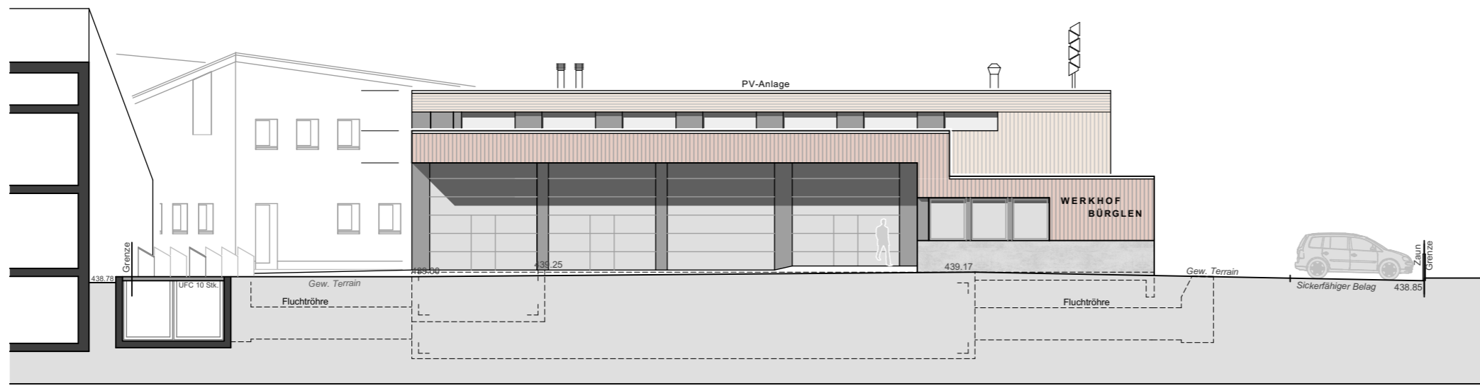
Nord-Westfassade
