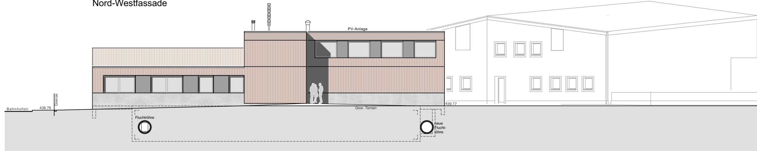
Süd-Westfassade
