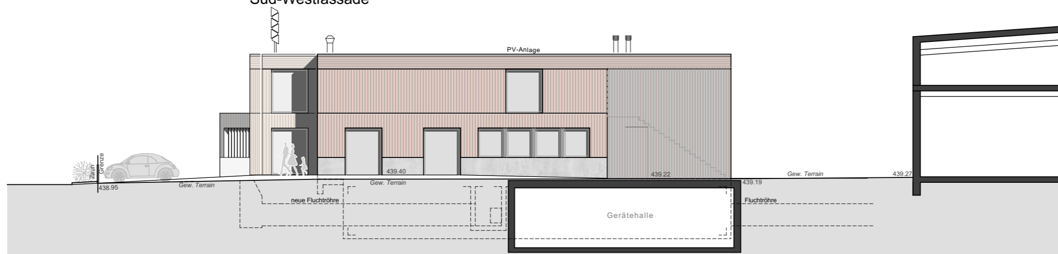
Süd-Ostfassade
