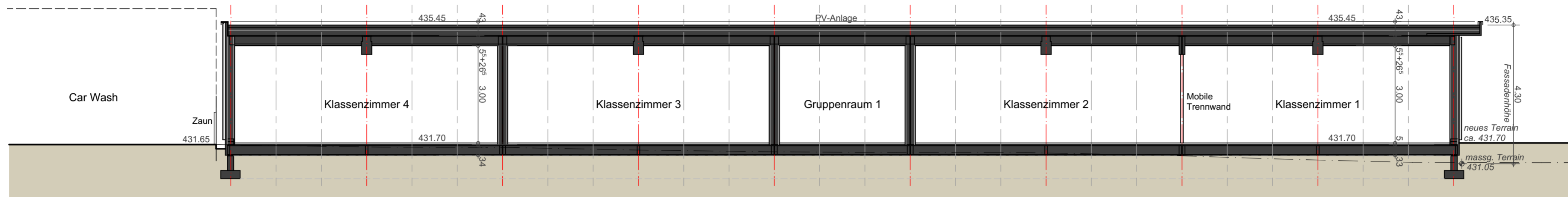
Längsschnitt
