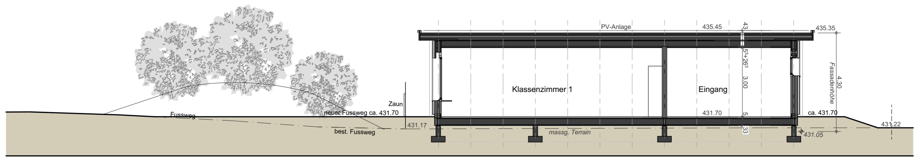
Querschnitt
