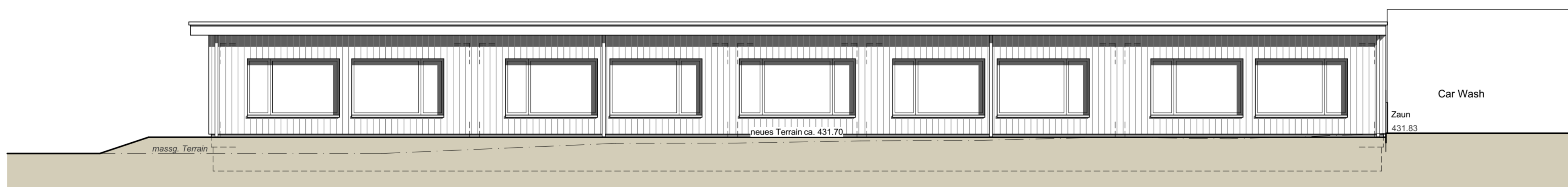
Nord-West Ansicht
