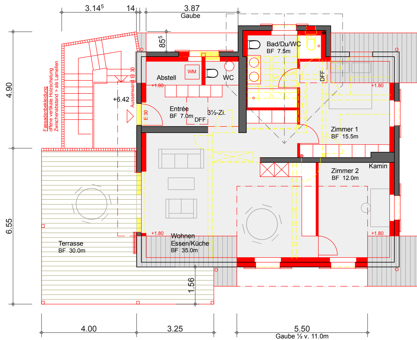
DACHGESCHOSS
